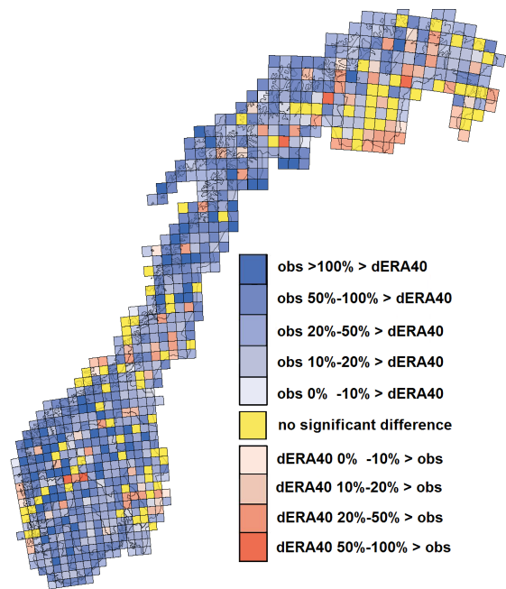
(d) Autumn; max blue: OBS 280% > dERA40, max red: dERA40 72% > obs.
